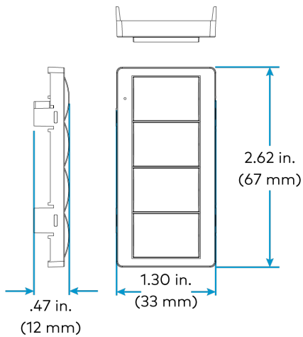
ZUMLINK-BTN4 (BLANK shown)
