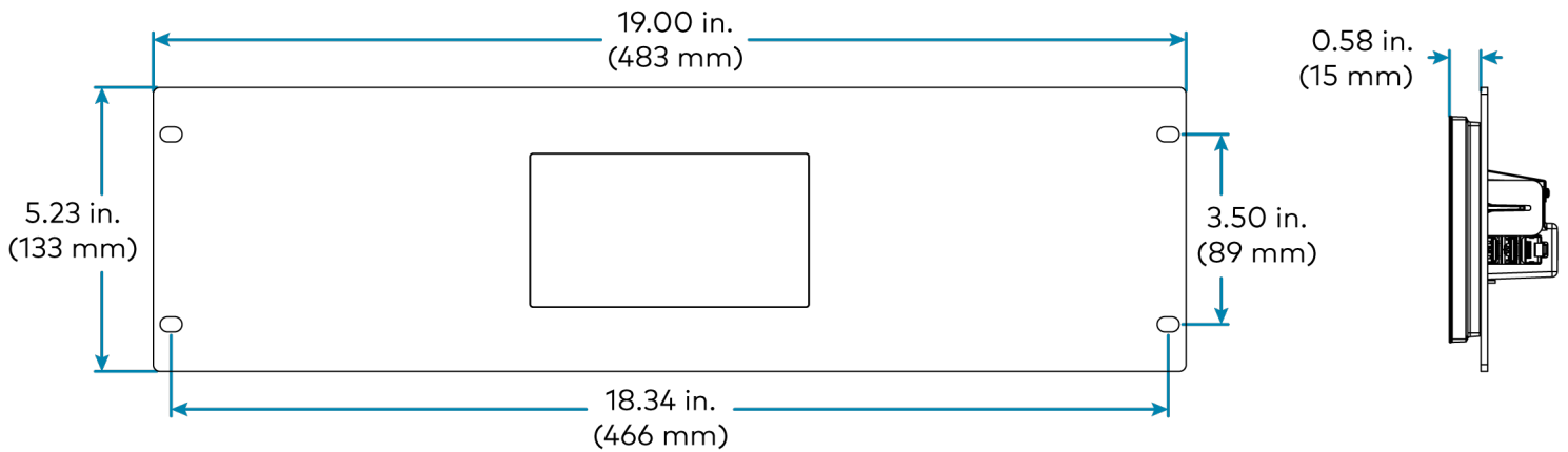
TSW-570/770-RMK-1 with TSW-770
