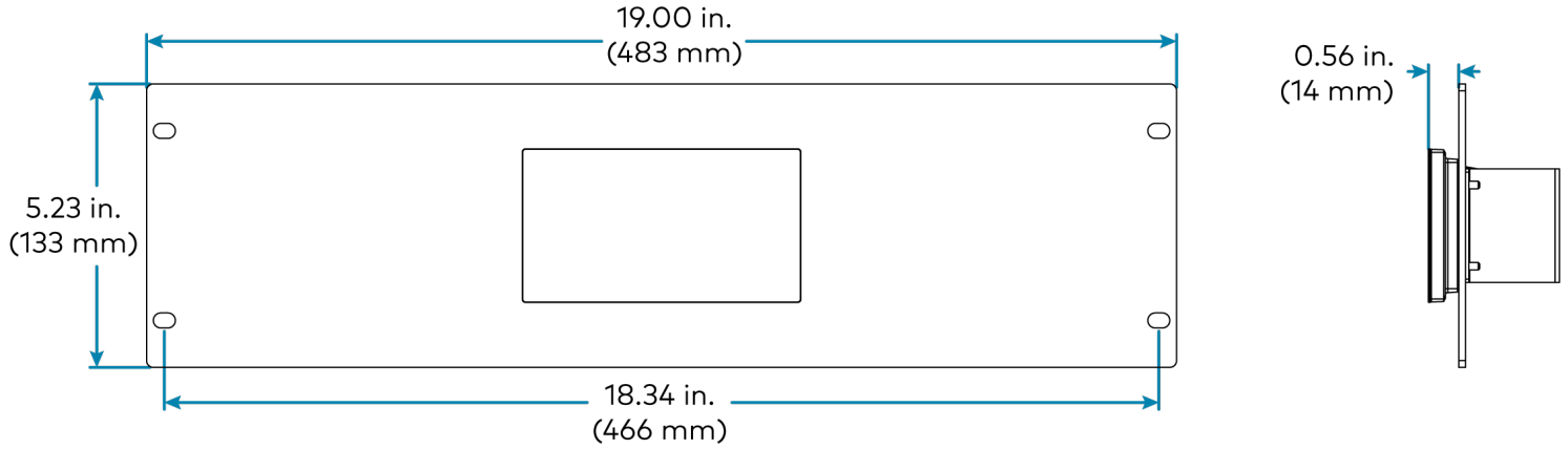
TSW-570/770-RMK-1 with TSW-570
